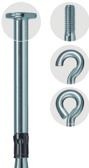
Strop podwieszany
