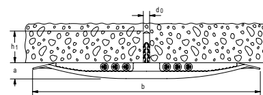
Zacisk wtykowy ClipFix SF z wieszakiem kablowym SF plus KB 16
