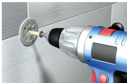
Wkręcanie kołków do płyt izolacyjnych
