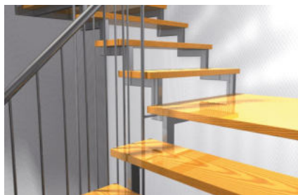
Mocowanie stopnic na schodach metalowych
