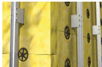
Termoizolacja w fasadzie wentylowanej
