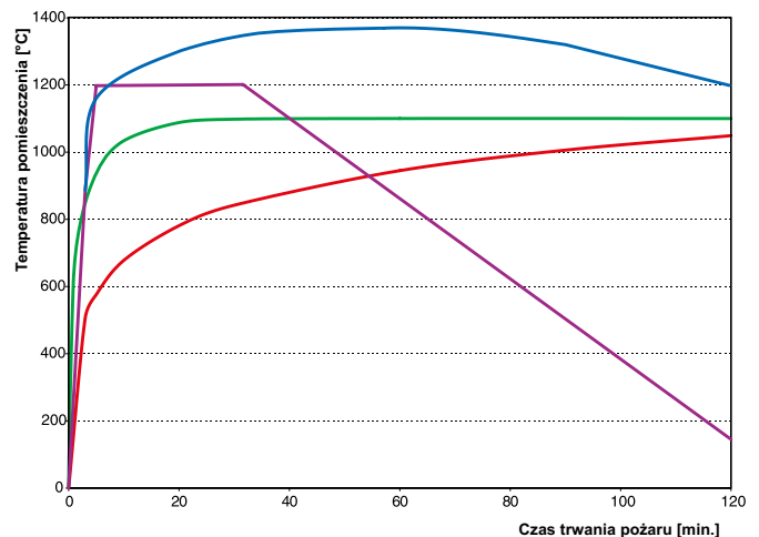
Krzywe temperaturowe: — (ETK) — krzywa węglowodorowa — AABT/ZTV krzywa tunelowa — krzywa Rijkswaterstaat tunnel
