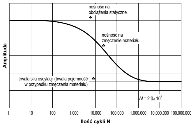
Krzywa Woehlera
