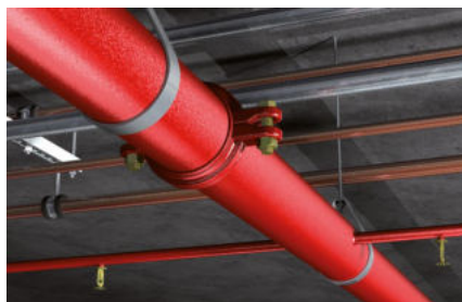
Instalacje tryskaczowe
