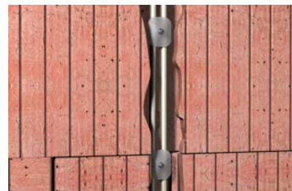
Mocowanie kabli w szczelinach
