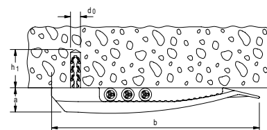
Zacisk wtykowy ClipFix SF z wieszakiem kablowym SF plus KB 8
