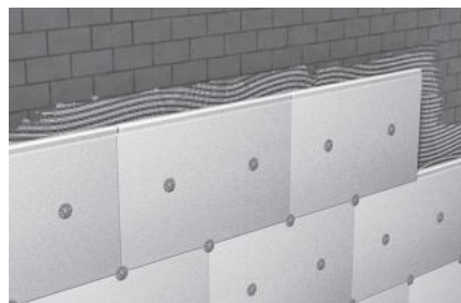
Sztywne płyty styropianowe O35 na bloczkach silikatowych
