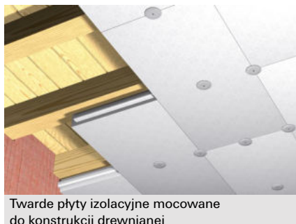
Twarde płyty izolacyjne mocowane do konstrukcji drewnianej
